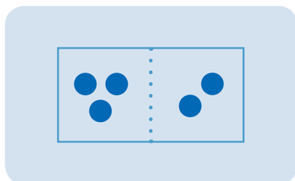
Abbildung 7: Teile-Ganzes-Konzept
