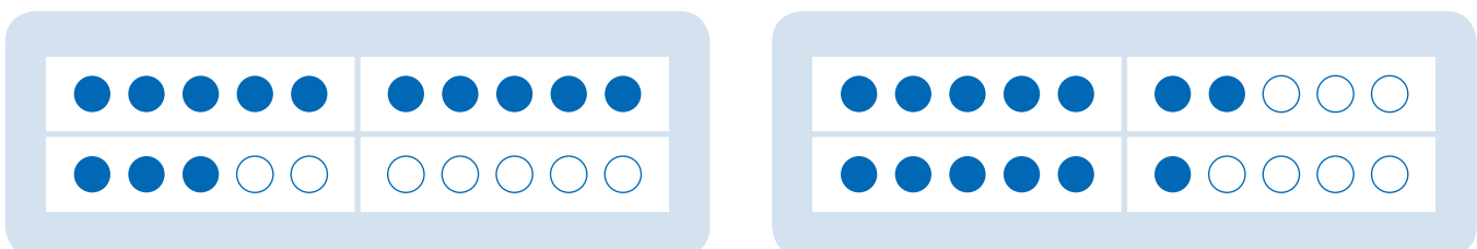
Abbildung 6: Darstellung der 13 am Zwanzigerfeld in Zeilendarstellung (links) und Blockdarstellung (rechts)
